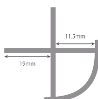
B. Außeneckprofil
