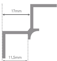
A. Inneneckprofil
